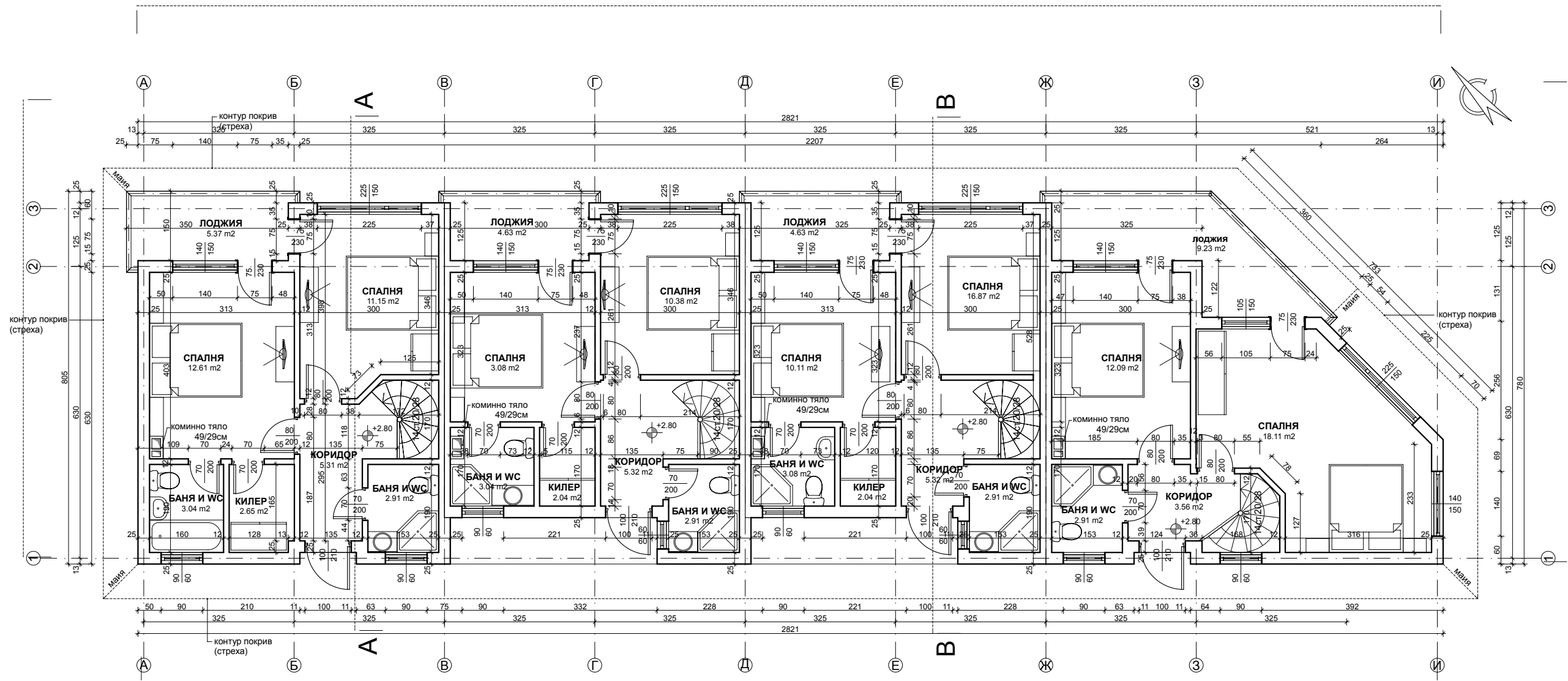
РАЗПРЕДЕЛЕНИЕ ВТОРИ ЕТАЖ КОТА +2,80; М 1:50 ЗП: 202.46 m 2
